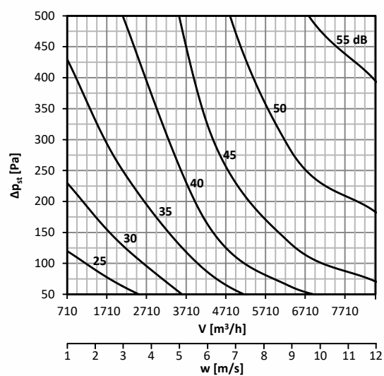
График 44. Уровень акустической мощности L_{WA} [дБ(A)], излучаемой мимо воздуховод DN500, с изоляцией
