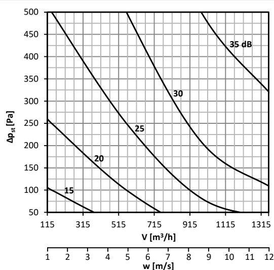
График 39. Уровень акустической мощности LWA [дБ(A)], излучаемой мимо воздуховод DN250, с изоляцией
