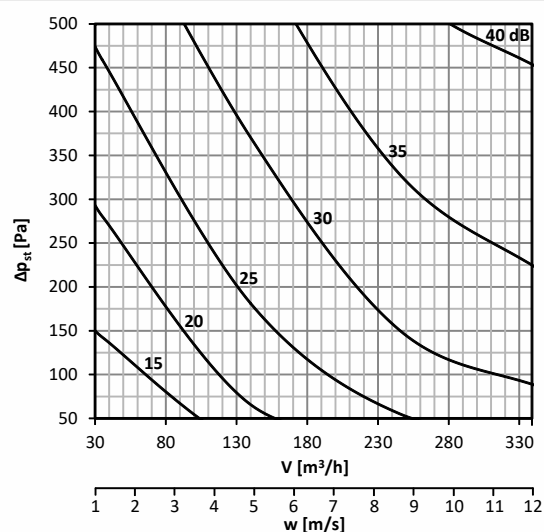
График 34. Уровень акустической мощности L_{WA} [дБ(A)], излучаемой мимо воздуховод DN140, с изоляцией
