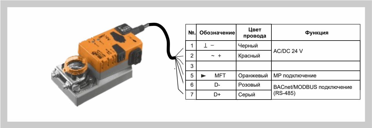
Рис. 9 Сервоприводы LMV-D3-MOD и NMV-D3-MOD
