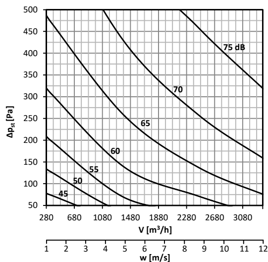
График 11. Уровень акустической мощности LWA [дБ(A)], выделяемой в воздуховод DN315
