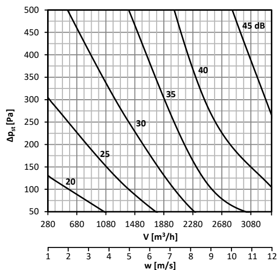
График 41. Уровень акустической мощности LWA [дБ(A)], излучаемой мимо воздуховод DN315, с изоляцией
