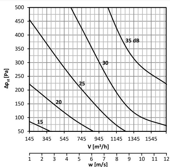
График 40. Уровень акустической мощности LWA [дБ(A)], излучаемой мимо воздуховод DN280, с изоляцией
