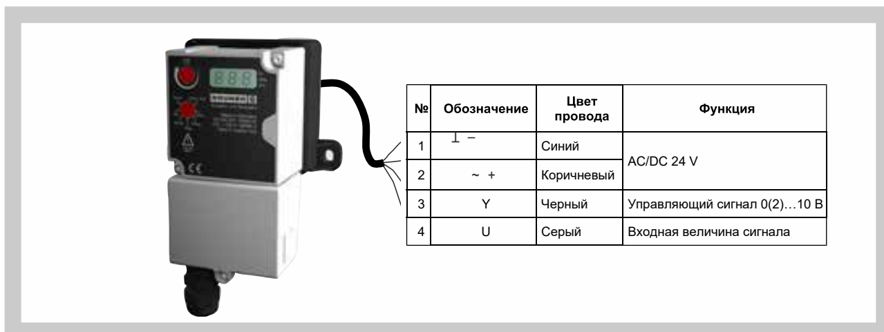
Рис.18 Регулировка GUAC-...
