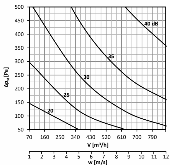
График 35. Уровень акустической мощности L_{WA} [дБ(A)], излучаемой мимо воздуховод DN160, с изоляцией
