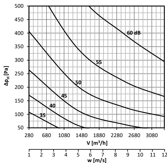
График 26. Уровень акустической мощности LWA [дБ(A)], излучаемой мимо воздуховод DN315, без изоляции
