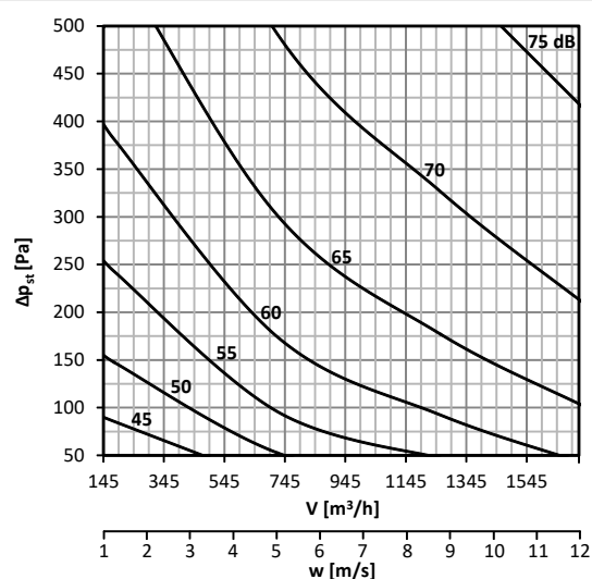
График 10. Уровень акустической мощности LWA [дБ(A)], выделяемой в воздуховод DN280
