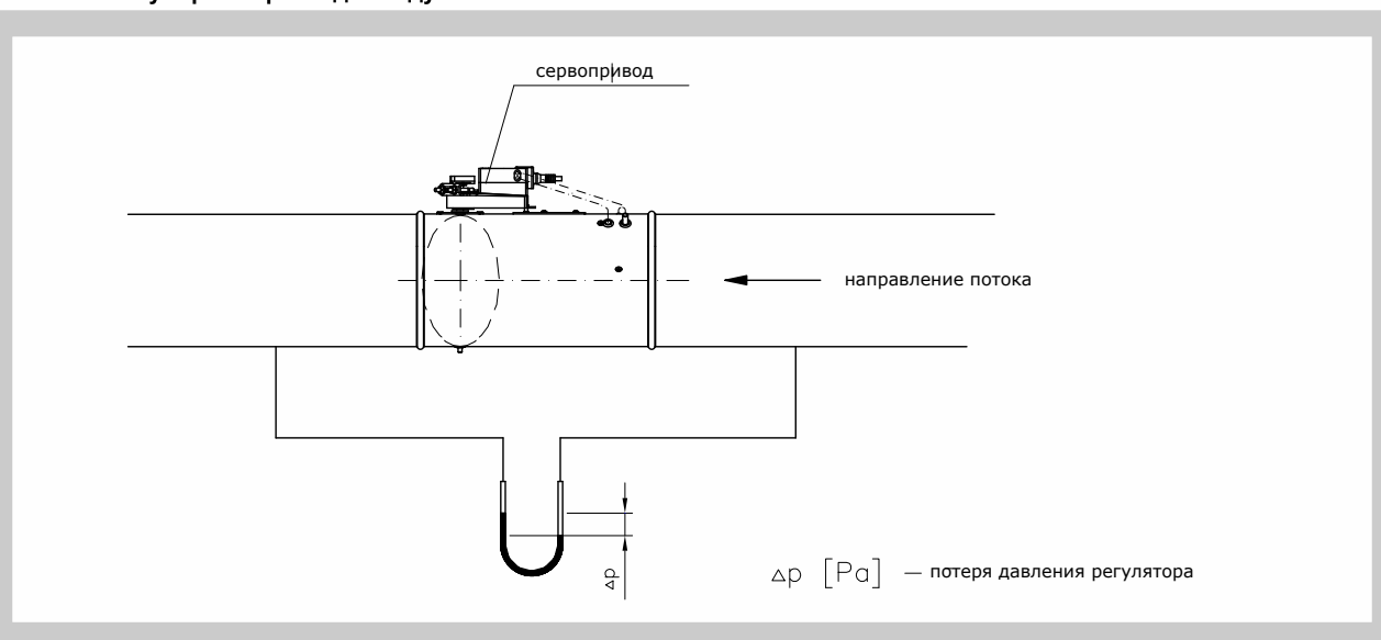
Рис. 4 Регулировка давления в воздуховоде
