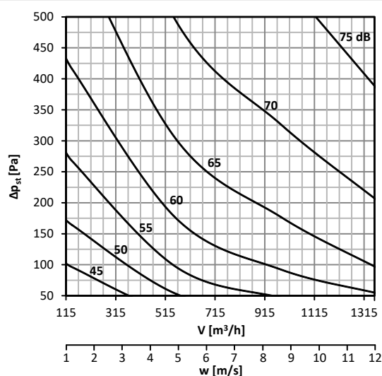
График 9. Уровень акустической мощности LWA [дБ(A)], выделяемой в воздуховод DN250
