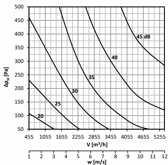
График 45. Уровень акустической мощности L_{WA} [дБ(A)], излучаемой мимо воздуховод DN630, с изоляцией
