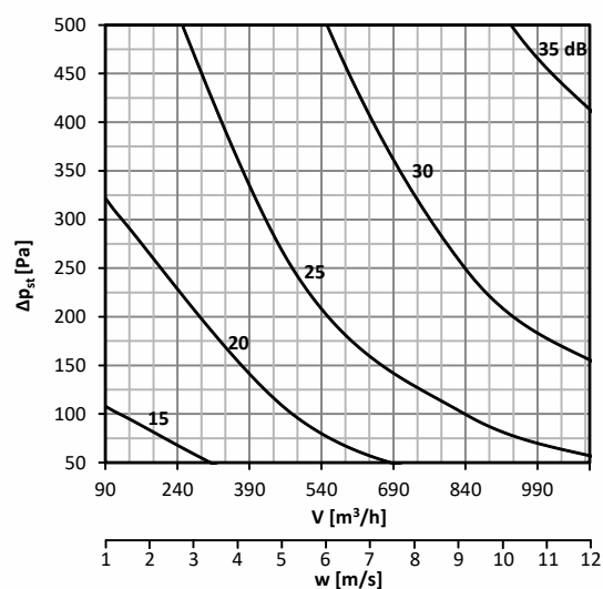
График 36. Уровень акустической мощности L_{WA} [дБ(A)], излучаемой мимо воздуховод DN180, с изоляцией
