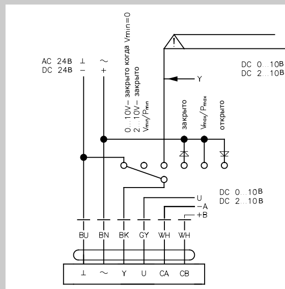
Рис. 20 Регулятор GUAC-...-MP
