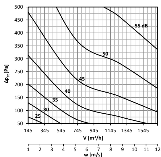
График 25. Уровень акустической мощности LWA [дБ(A)], излучаемой мимо воздуховод DN280, без изоляции
