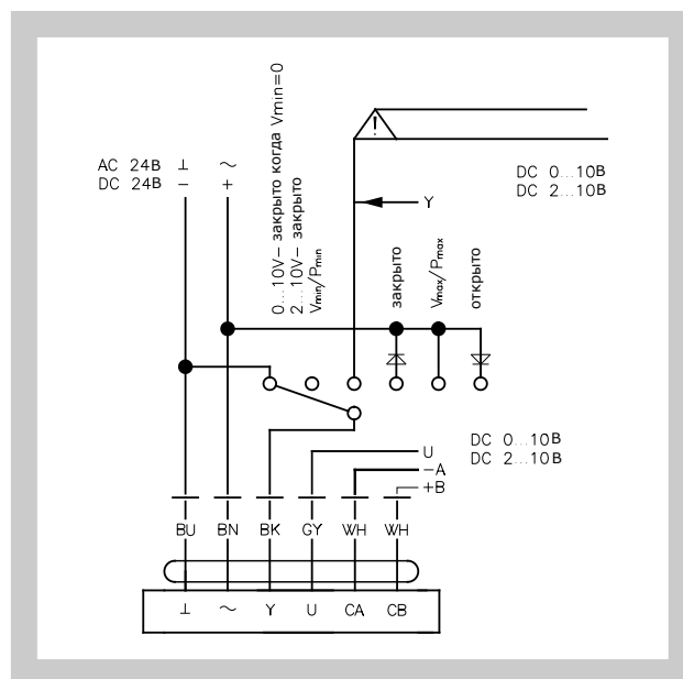
Рис. 17 Регулировка 227VM-024-...-MP и 227PM-024-...-MP
