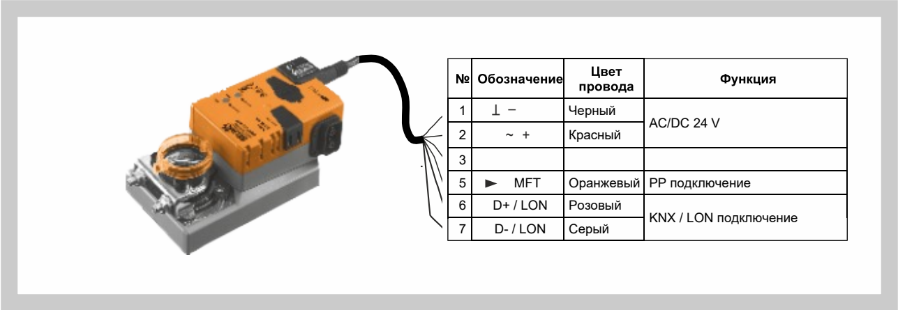
Рис. 13 Подключение сервоприводов LMV-D3-LON и NMV-D3-LON
