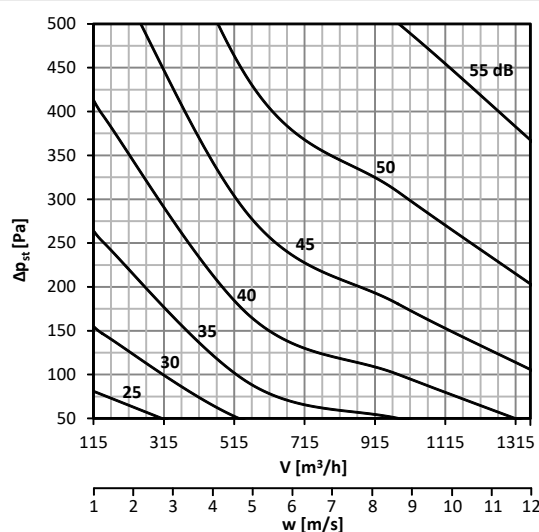
График 24. Уровень акустической мощности LWA [дБ(A)], излучаемой мимо воздуховод DN250, без изоляции
